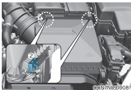
3. 에어클리너 필터를 앞으로 당겨 교체하십시오.
