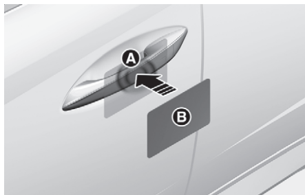
[A] 도어 핸들 인증 패드 [B] 카드 키 NFC 안테나
