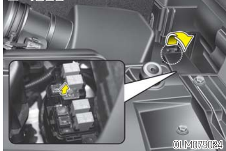
■ 디젤엔진
