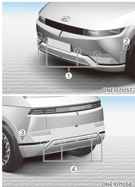
[1]: 전방 초음파센서, [2]: 전측방 초음파센서 [3]: 후측방 초음파센서, [4]: 후방 초음파센서
