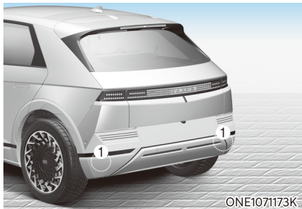
[1]: 후측방 레이더
