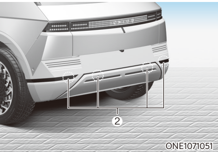
[1]: 전방 초음파센서, [2]: 후방 초음파센서
