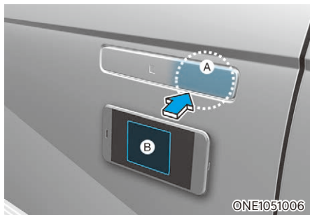
[A]: 도어 핸들 인증 패드 [B]: 스마트폰 뒷면에 있는 NFC 안테나 (스마트폰마다 위치 다름)
