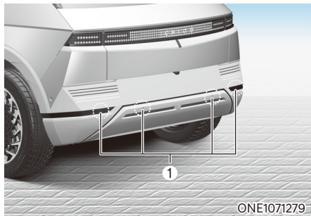
[1]: 후방 초음파센서
