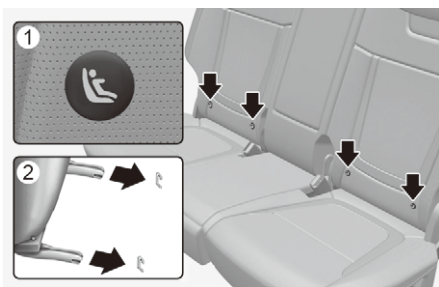
(1) 로어 앵커 심볼
