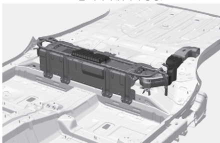
고전압 배터리(뒷좌석 중앙)
