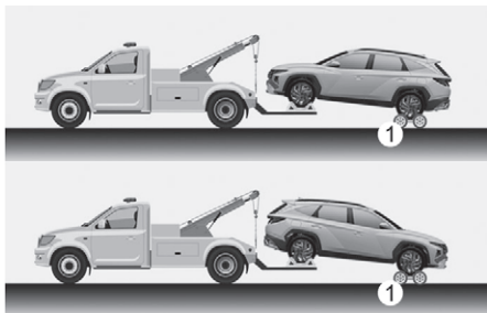
타이어 구속 견인
